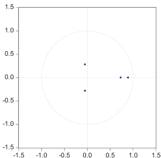
Figura 2. Raízes inversas do polinômio característico
